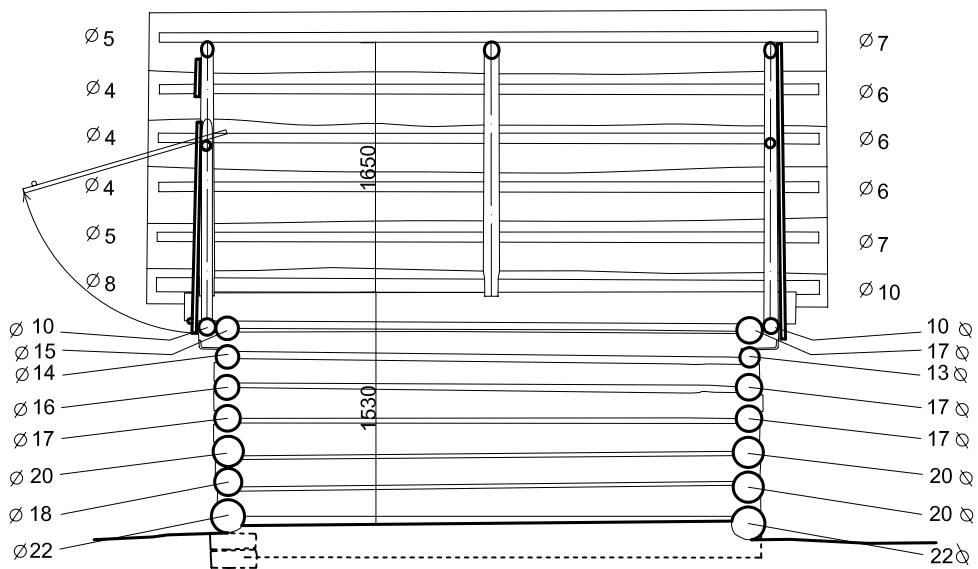
Rez BB
