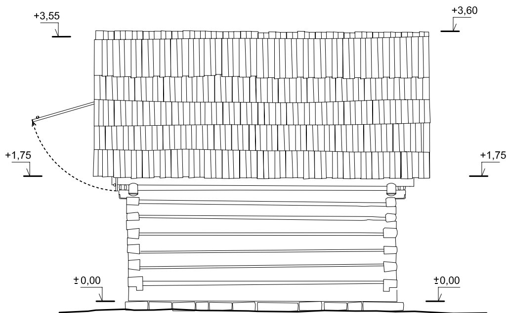
Pohľad severný
