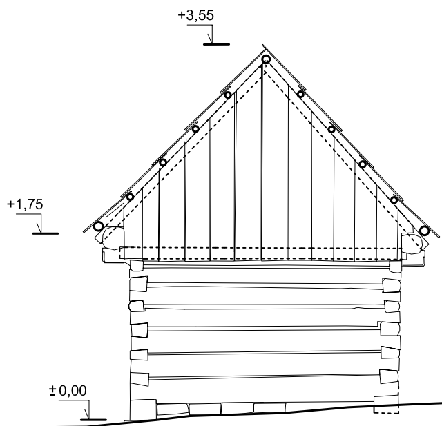
Pohľad západný
