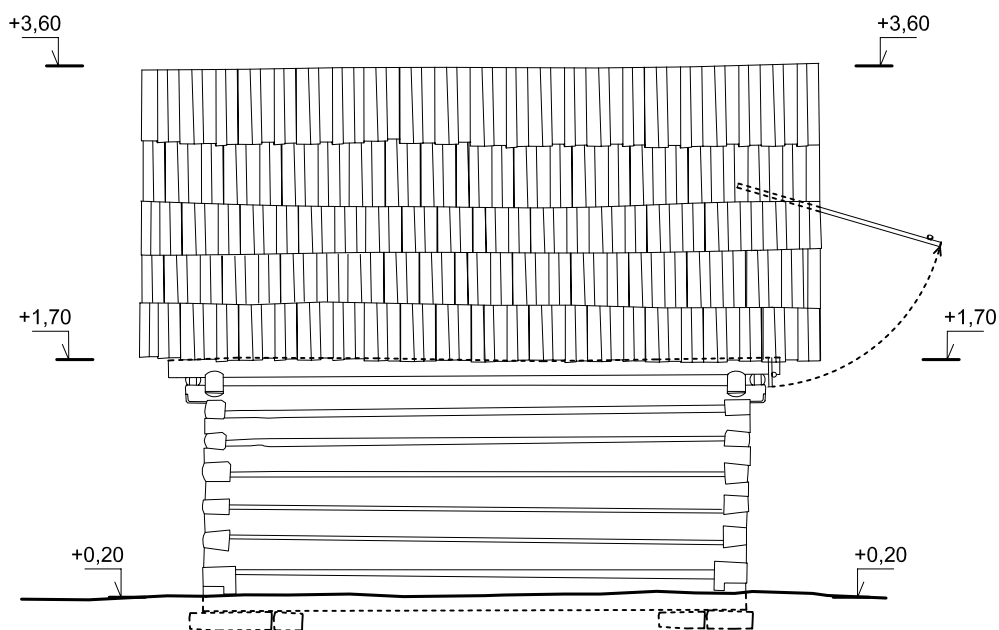
Pohľad južný
