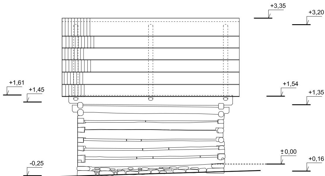
Pohľad Západný
