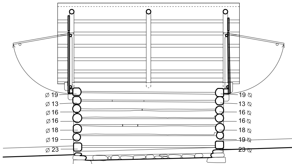
Rez BB
