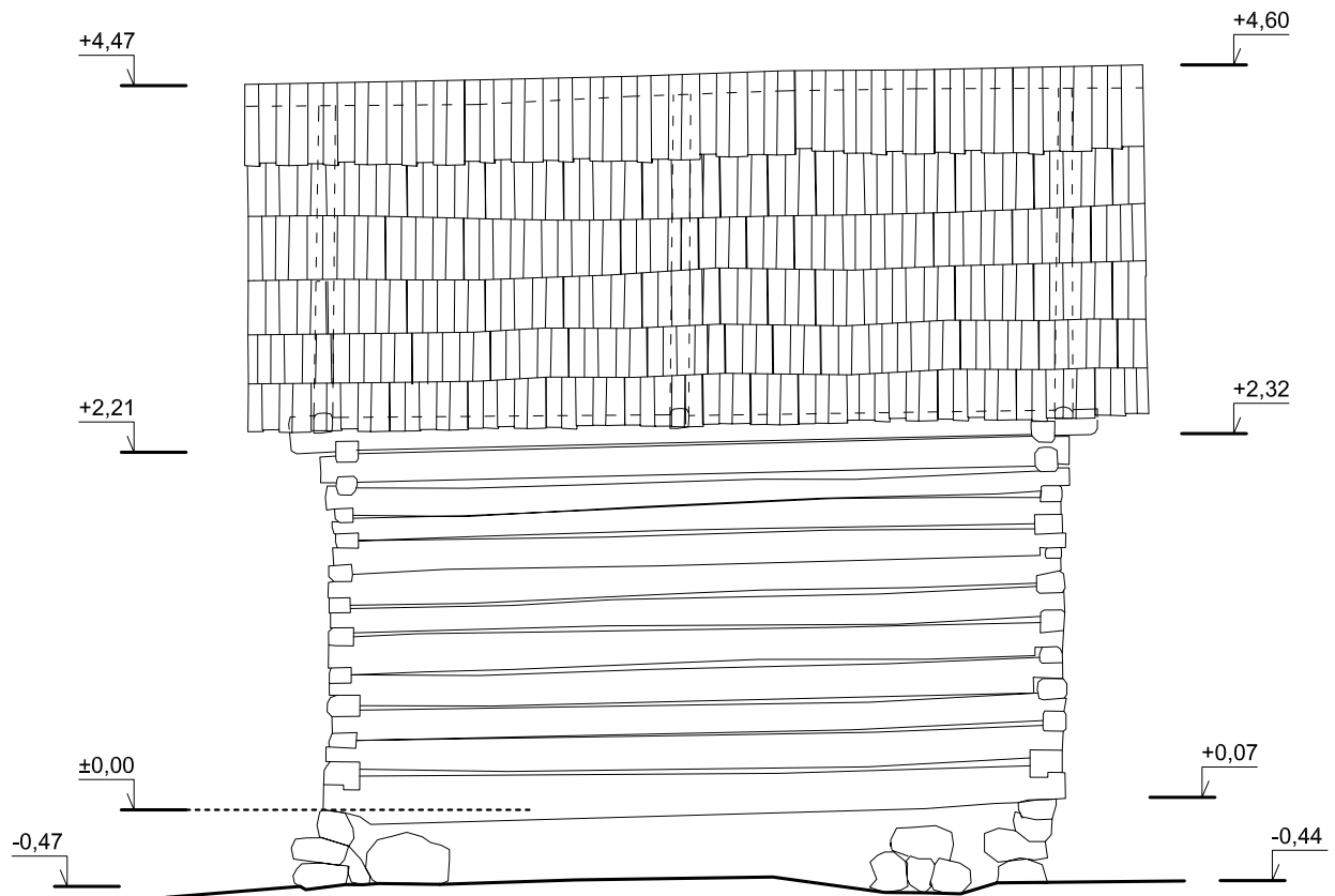
Pohľad južný
