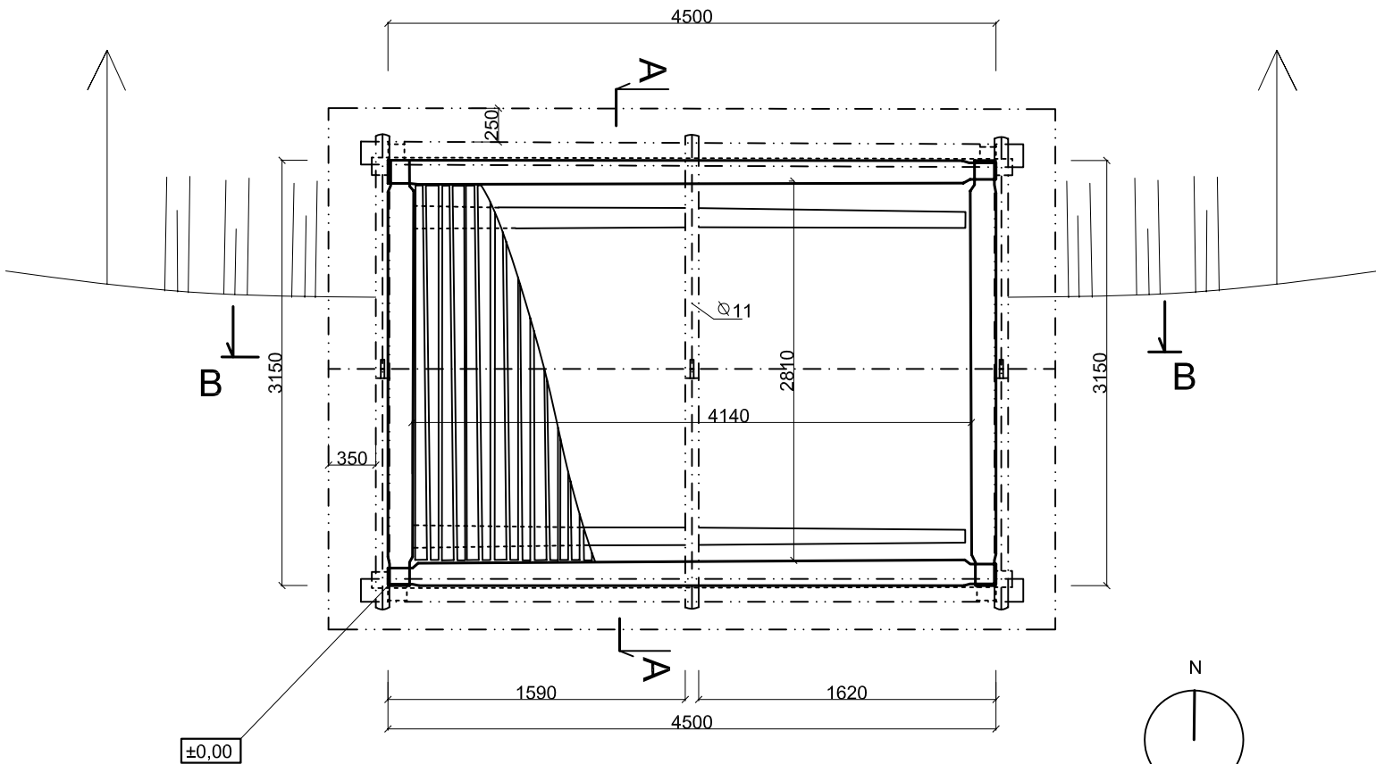
Pôdorys_S10
