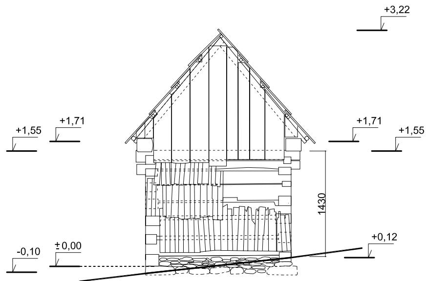
Pohľad severozápad
